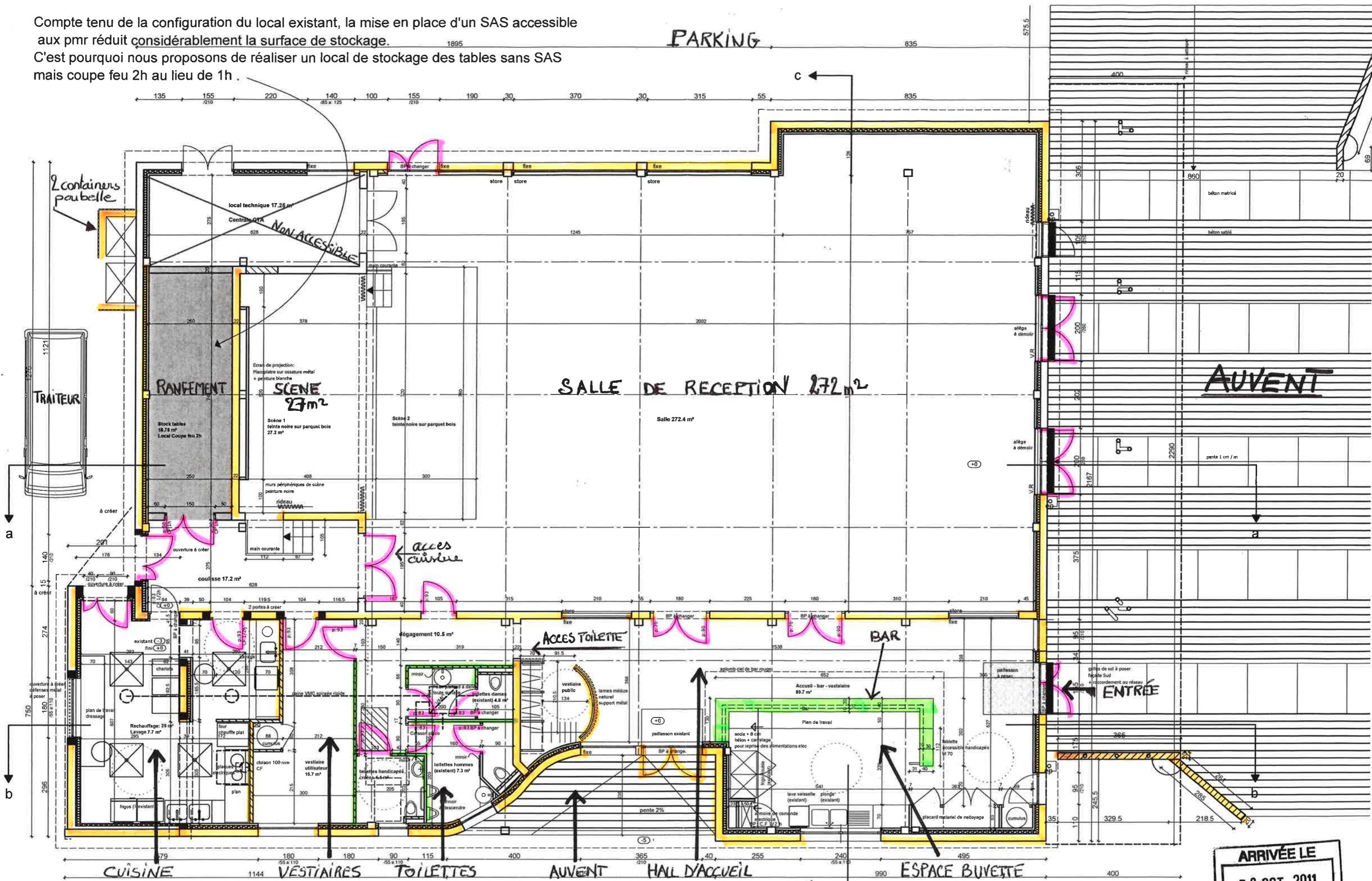
Plan Projet 1/100
